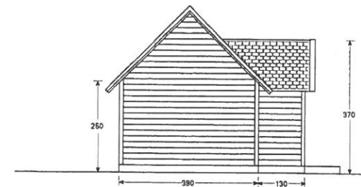
FASAD MOT VÄST
