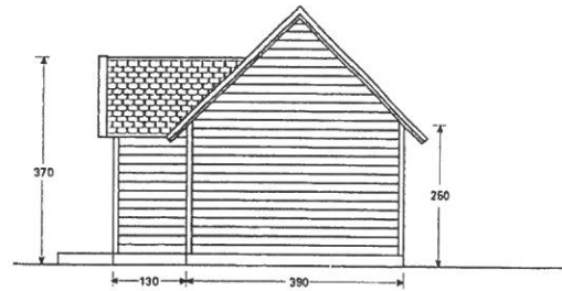
FASAD MOT ÖST
