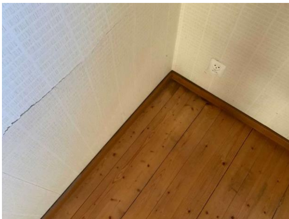
Bild 20: Invändigt, Källarplan, Gillestuga + sovrum, Uppbyggda golv med fuktskador samt fuktfläckar på tapeter se fortsatt teknisk utredning
