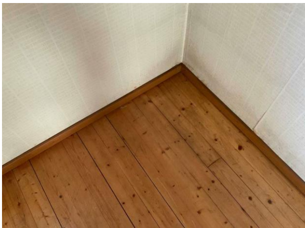
Bild 19: Invändigt, Källarplan, Gillestuga + sovrum, Uppbyggda golv med fuktskador samt fuktfläckar på tapeter se fortsatt teknisk utredning
