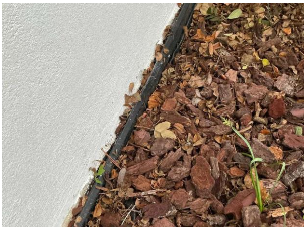
Bild 1: - Utvändigt, Grundmur/Hussockel, Topplist mot platonmatta ej tät mot grundmuren vatten kan tränga in bakom topplist
