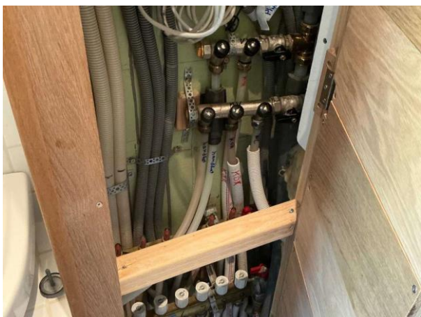
Bild 9: Invändigt, Plan 1, Tät botten saknas i inbyggnad för vattenkopplingar
