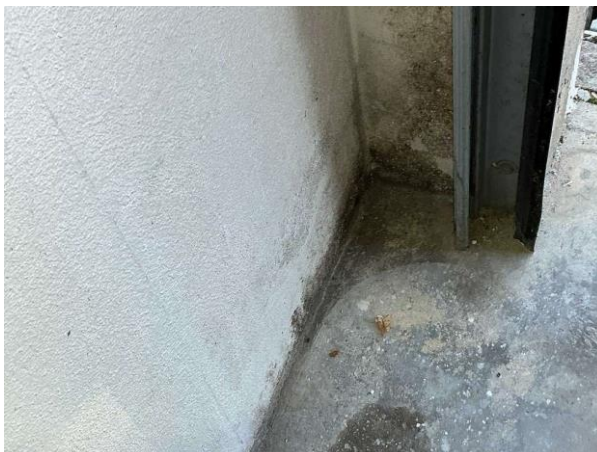
Bild 8: Invändigt, Garage, Fuktkänslighet noterades i källarväggs nedre kant
