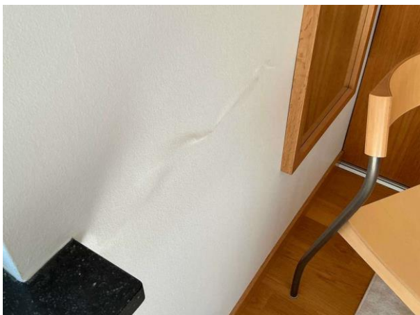
Bild 11: Invändigt, Plan 2, Bula på vägg vid fönster (det kan ha uppstått sprickor i bakomliggande vägg under tapet)
